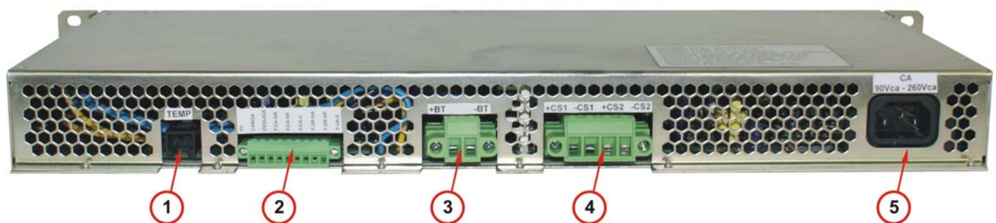
Figura 3 – Vista traseira.
