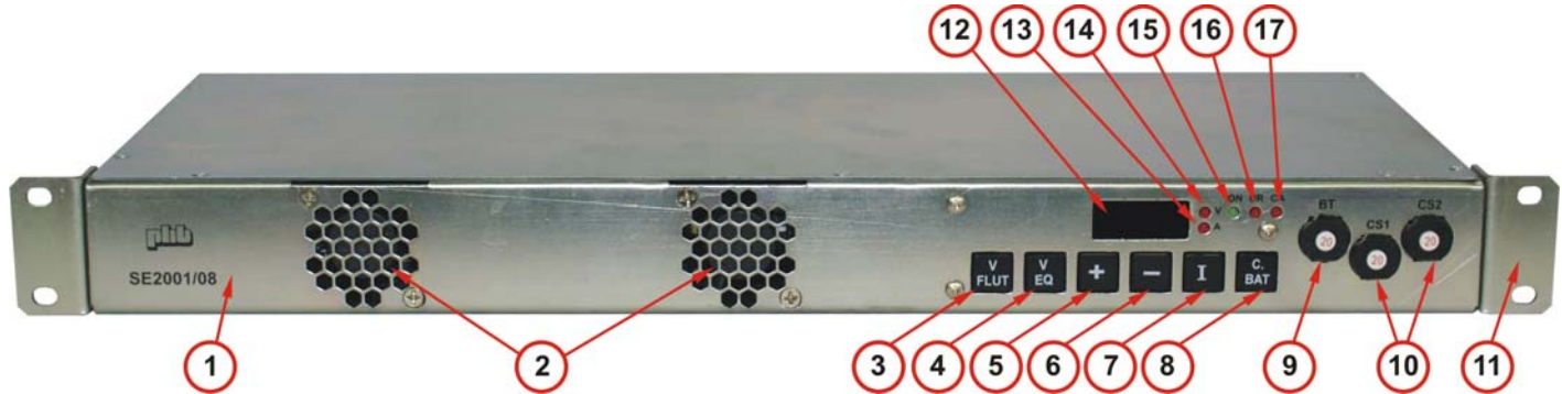
Figura 2 – Vista frontal.
