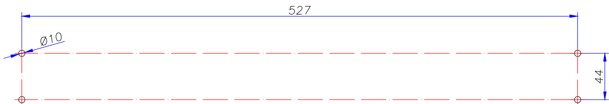
Figura 8 – Furação de parede (cotas em mm).
