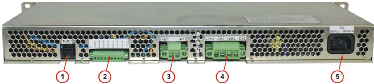
Figura 9 – Conexões elétricas.
